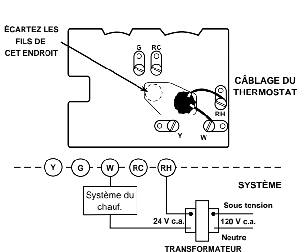
Figure 4. Chauffage seulement à 2 fils et un transformateur
