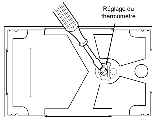
Arrière du couvercle du thermostat
