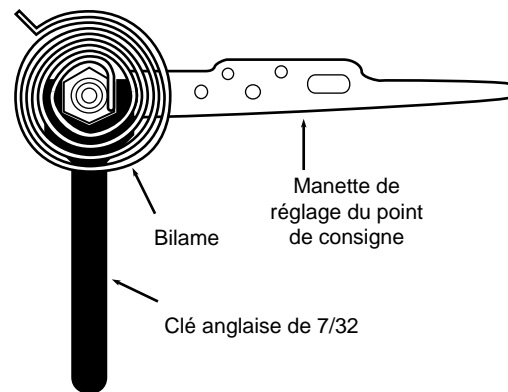
Figure 12. Étalonage du thermostat
