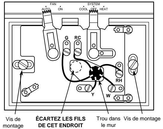
Figure 2. Socle du thermostat
